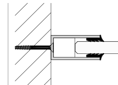
Wandanschluss gerade
