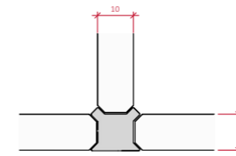
T - Profil ESG 10mm
