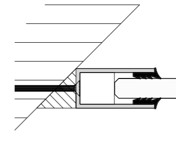
Wandanschluss 45°
