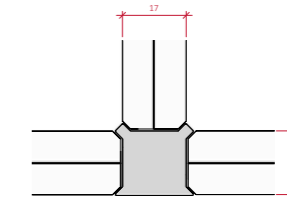
T - Profil VSG 17mm
