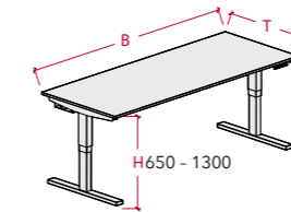
T-Fuß, 2-fach teleskopierbar
