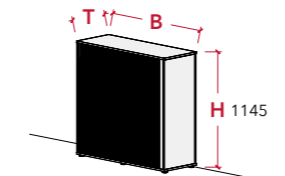
Querrolladenschrank 3 OH 2 Fachboden verstellbar
