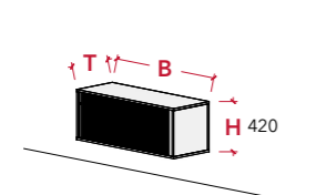
Querrolladenschrank 1 OH
