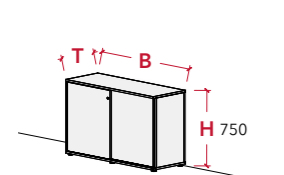
Schiebetürenschränk 2 OH 1 Fachboden verstellbar
